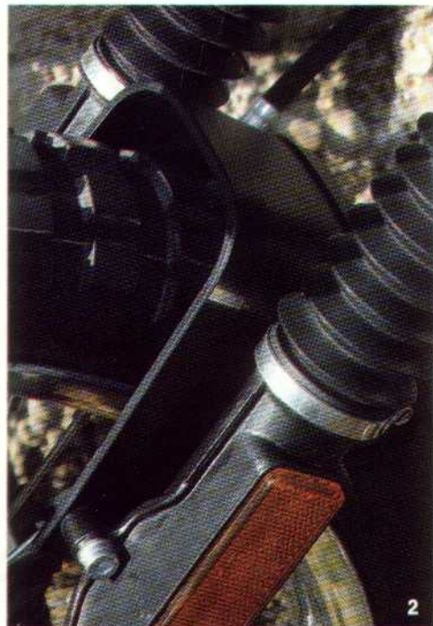
(2) Il rinforzo forcella telescopica BMW conferisce maggiore rigidità alla forcella.
