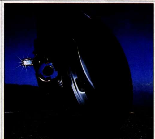
Starke Optik mit Effekt. Leichtmetallfelgen mit 3-Speichen im U-Profil zur Verringerung der ungefederten Massen und Niederquerschnittreifen in den Dimensionen 120/70 VR 17 vorn und 160/60 VR 18 hinten für bessere Bodenhaftung vor allem bei Schräglage. Ebenfalls neu: 4in1-Edelstahlauspuffanlage mit rundem Endschalldämpfer.
